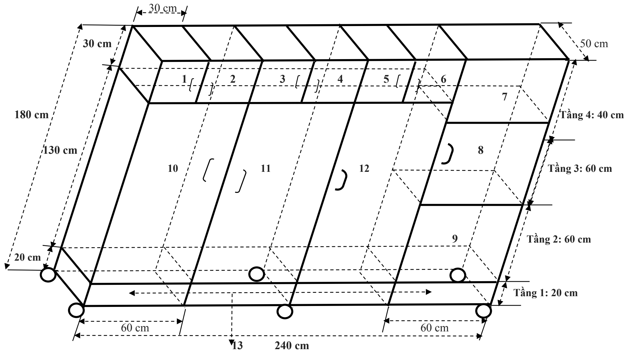
BẢNG VẼ TỦ GỖ ĐỂ QUẦN ÁO PHẪU THUẬT VIÊN
